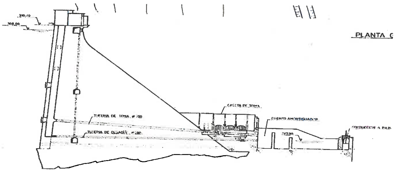
PERFIL LONGITUDINAL DEL APROVECHAMIENTO Esc 1:250
